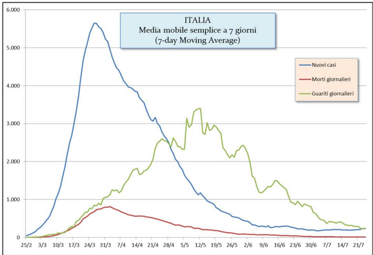
Figura 2 - Media mobile semplice a 7 giorni
