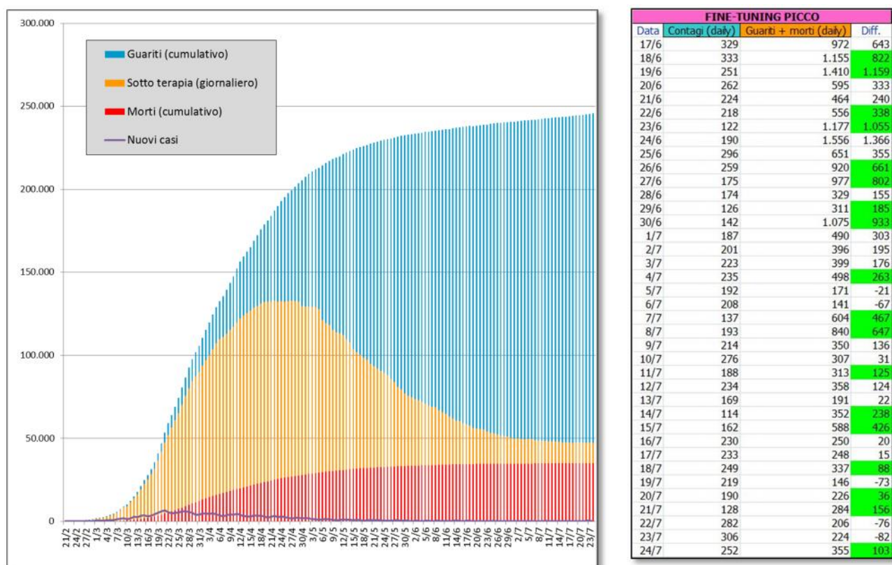
Figura 1 - Curva dei sotto terapia (in arancio) e dati relativi
